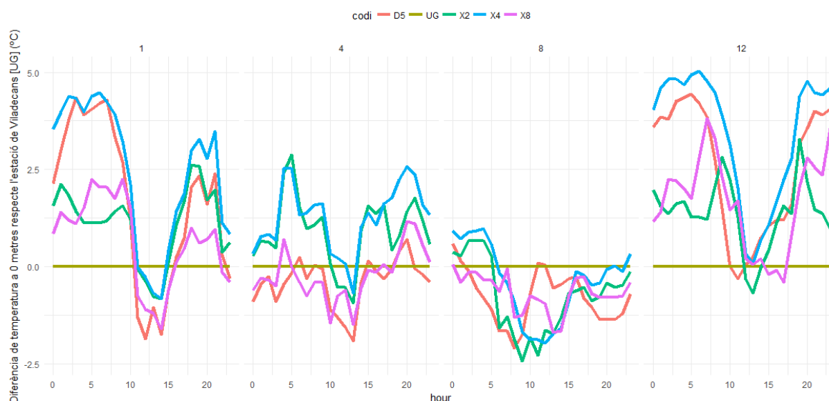
Gràfic 5: Exemple de la diferència de la temperatura a 0 metres d'alçada respecte l'estació de Viladecans [UG] del dia 1 de gener, abril, agost i desembre de 2016
