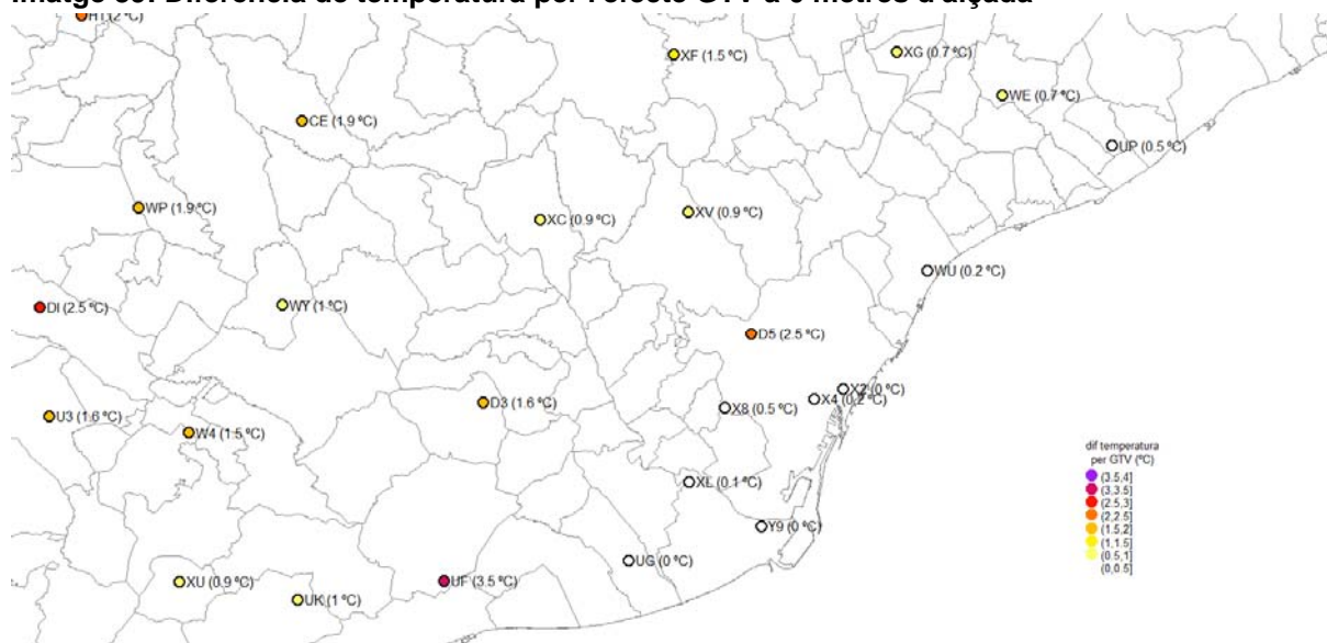
Imatge 39: Diferència de temperatura per l'efecte GTV a 0 metres d'alçada
