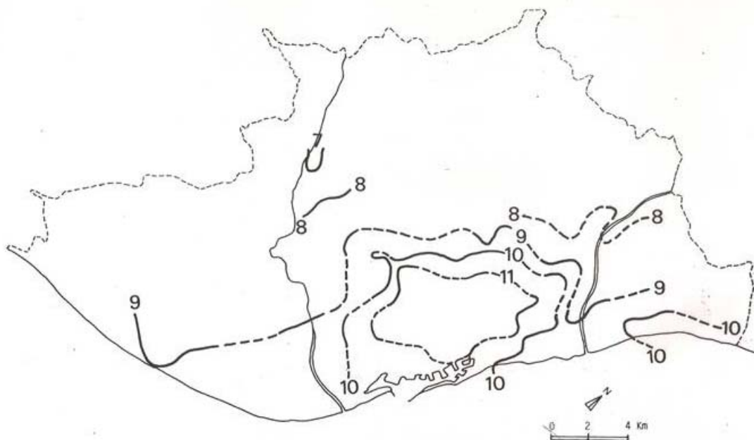
Imatge 30. Isothermes (en °C) de 26/10/1986 23.05h de l'AMB
